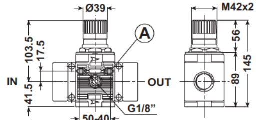
A FORI DI FISSAGGIO Ø 5.5 FIXING HOLES Ø 5.5
